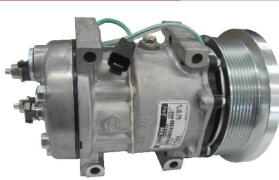
CP15166 COMPRESOR SD7H15HD 8 RANURAS 24 VOLTS (133MM) MONTAJE DIRECTO
